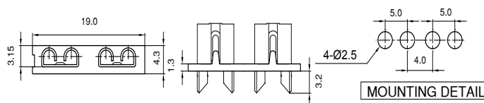
CQ-122 For AST Mini Blade Type Fuse
